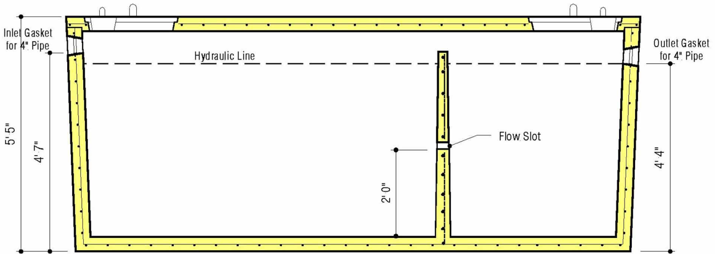
SECTION A-A
