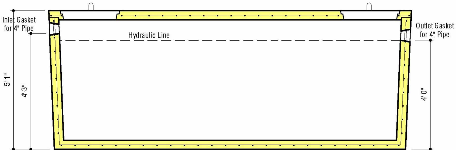
SECTION A-A
